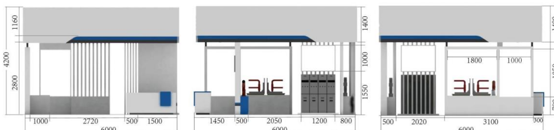
●立面图(单位mm)
